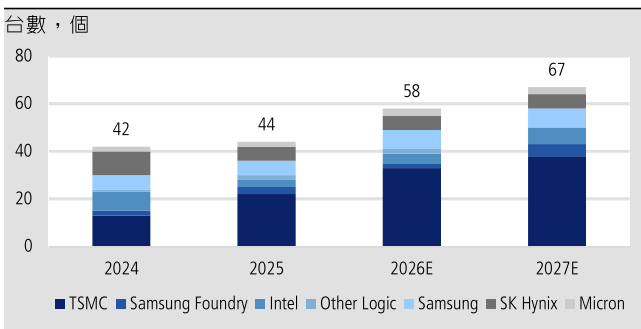
圖 5: Low NA EUV 機台出貨量預估
