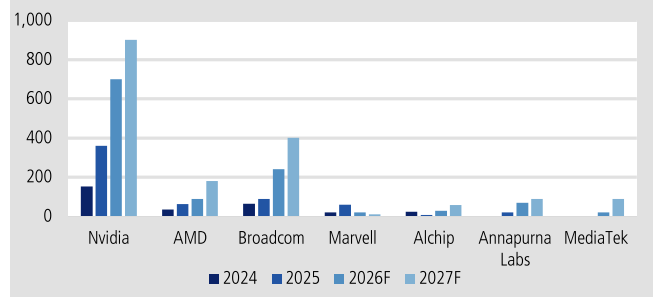
圖 6：2025-27 年 CoWoS 預估出貨量(依客戶別)
