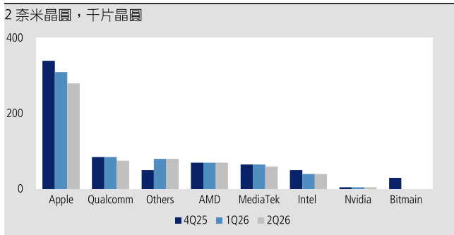
圖 3：台積電 N2 出貨預估變化 (依客戶)
