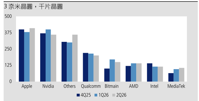
圖 4：台積電 N3 出貨預估變化 (依客戶)
