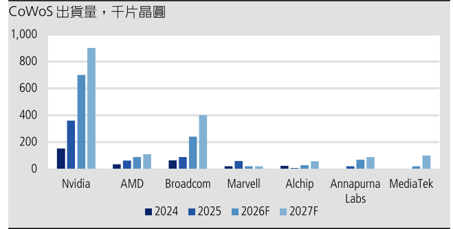
圖 2：2025-27 年 CoWoS 預估出貨量 (依客戶)
