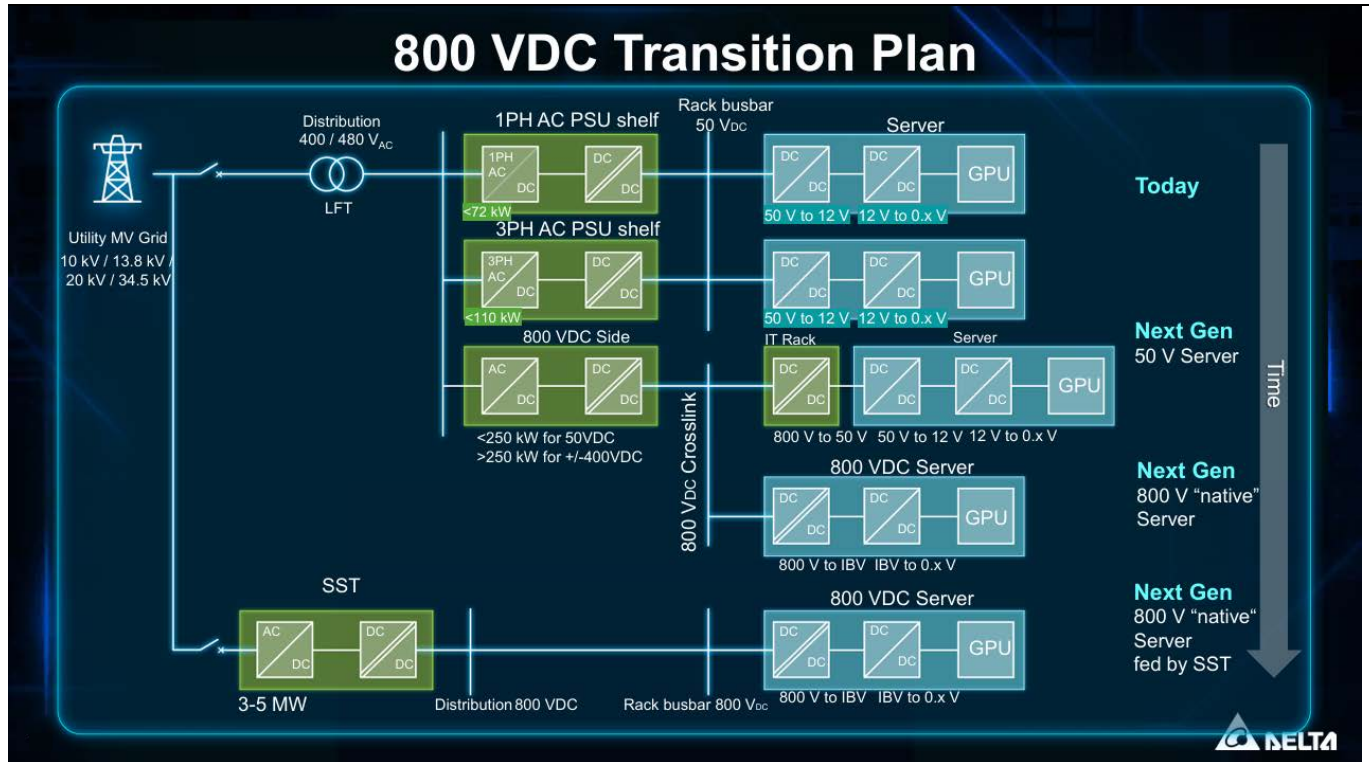
圖 7：台達電 HVDC 架構推進藍圖
