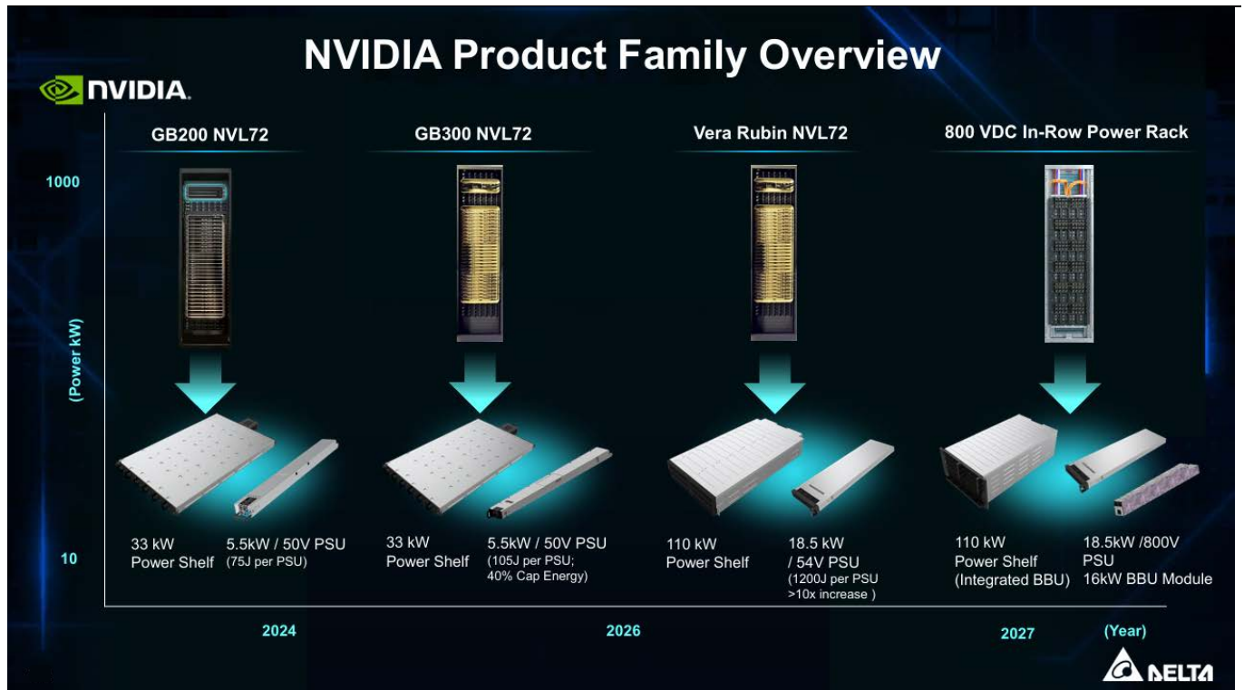
圖 8：台達電 PSU 產品在不同伺服器平台之規格
