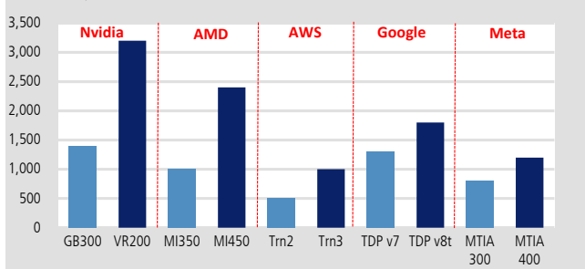
圖 4：AI 晶片熱設計功耗逐代提升，帶動水冷設計升級
