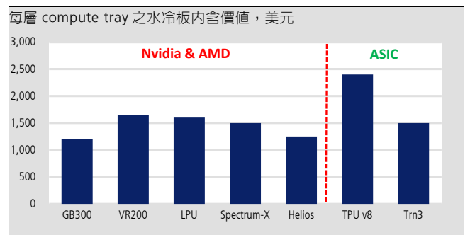
圖 5：迭代晶片推升晶片功耗，也拉升水冷板內含價值
