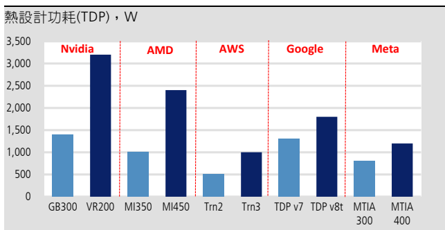
圖 4：AI 晶片熱設計功耗逐代提升；GPU 熱設計功耗始終高於 ASIC
