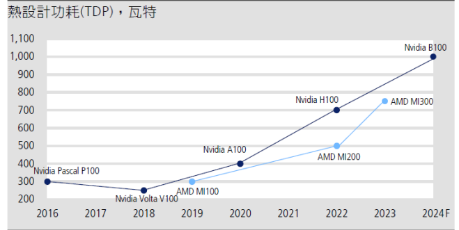
圖 5：GPU 之 TDP 較高
