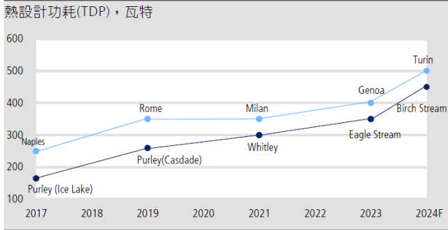
圖 4：伺服器 CPU TDP 逐年上升
